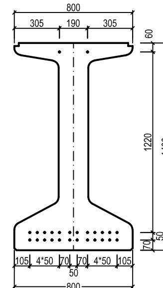
PRE DĹŽKU NOSNÍKA 27m (VP)
