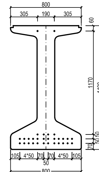
PRE DĹŽKU NOSNÍKA 30m (VP)
