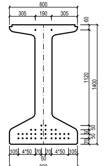
PRE DĹŽKU NOSNÍKA 32m (VP)
